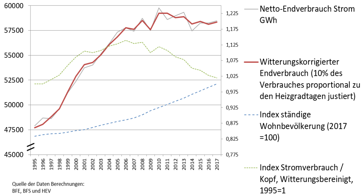
Endverbrauch Strom in der Schweiz 1995 bis 2017 (GWh)
